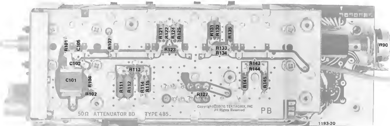
Fig. 8-1. A5 & A6 50 Ω Attenuator board.
